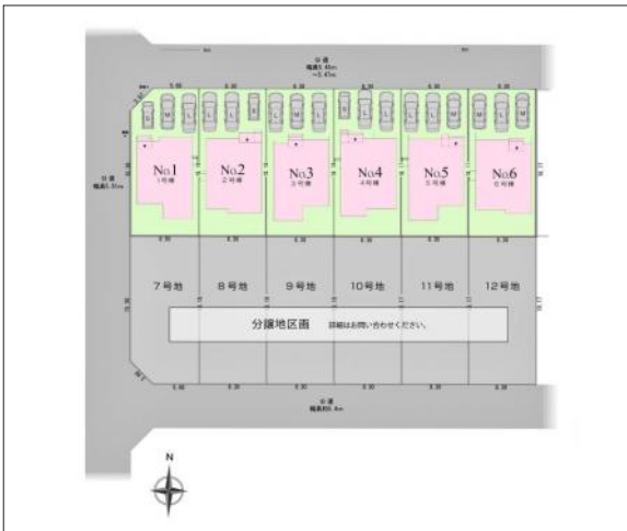
配置図
